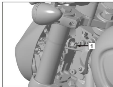
灯具调节螺丝
